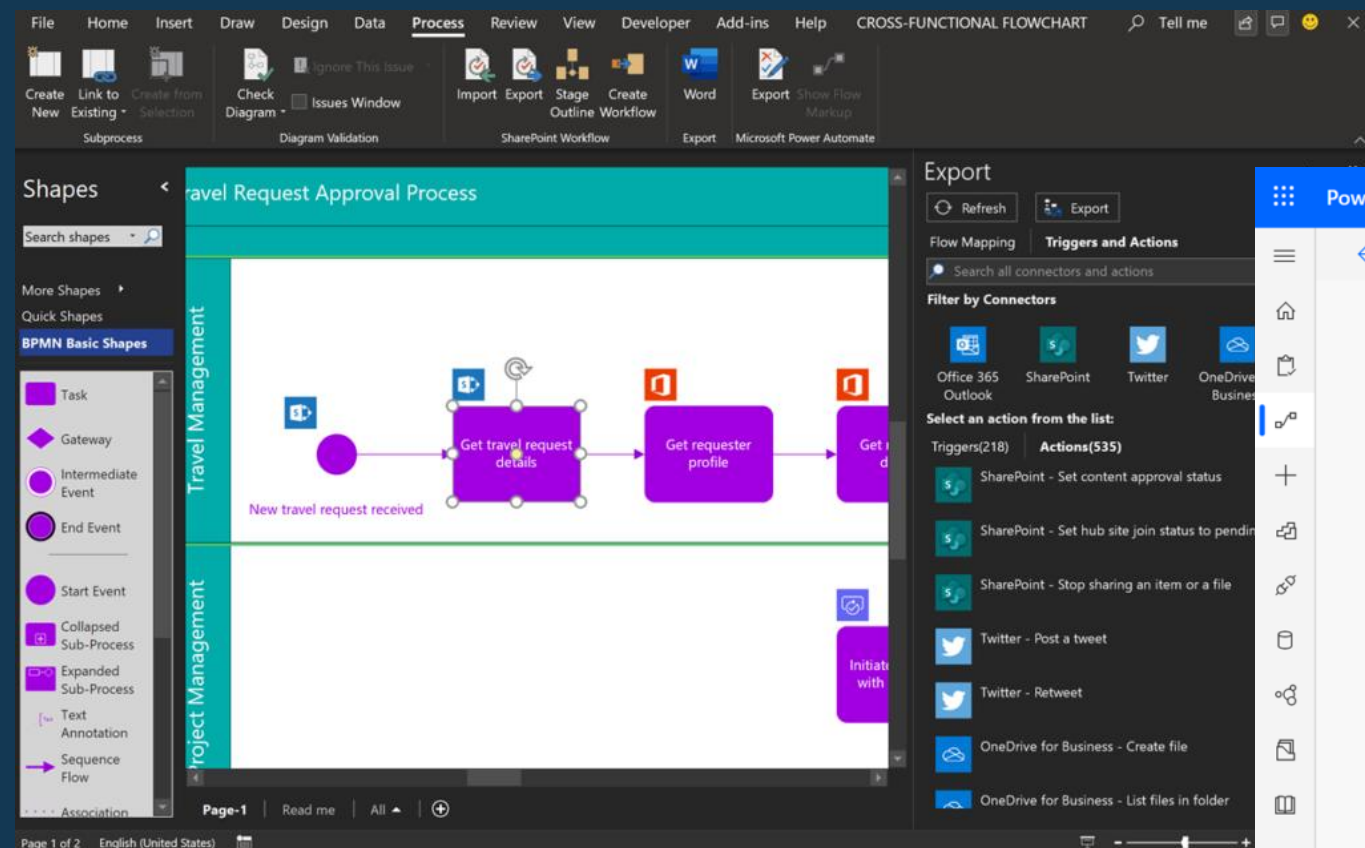
MS Visio
